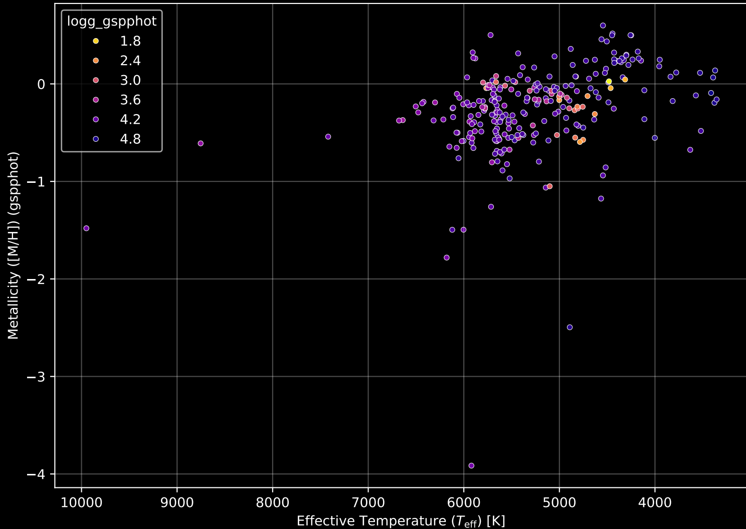
APOGEE DR17 Field: [sgr_tidal5] Stellar Population Parameters (n= 265)
